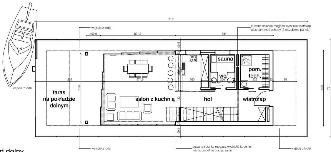
rzut - pokład dolny
